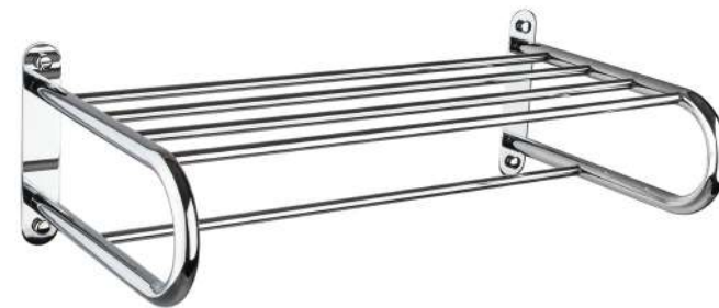
061500 Toallero repisa pletinas con barra 4 anclajes 50 cm. Acabado: cromo brillo. Material: latón. Towel shelf with bar 4 anchors 50 cm. Finish: bright chrome. Material: brass. 145 x 480 x 260 mm.
