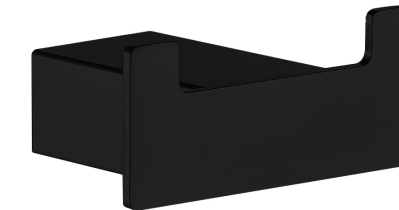
160002-N ●●●●● Percha doble KUO. Acabado: negro mate. Material: latón. Double robe hook KUO. Finish: matte black. Material: brass. 30 x 70 x 53 mm.
