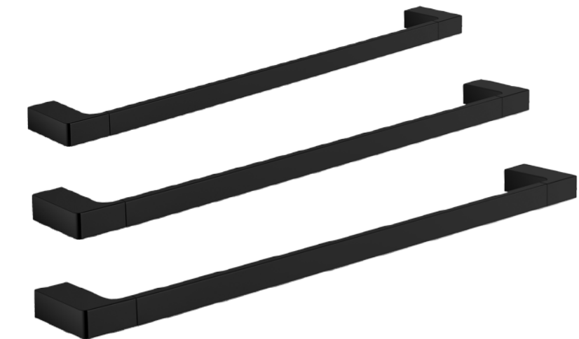
160300-N ●●●●● Toallero barra KUO 30 cm. Acabado: negro mate. Material: latón. Towel bar KUO 30 cm. Finish: matte black. Material: brass. 24 x 305 x 72 mm.
